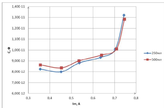
Рисунок 11 – Зависимость емкости механической ветви от тока механической ветви
