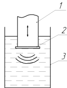
1 – волновод-концентратор; 2 – рабочий инструмент; 3 – технологический объем.
