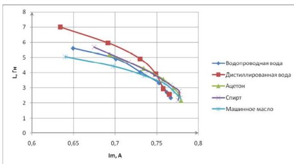
Рисунок 7 – Зависимость индуктивности механической ветви от тока механической ветви
