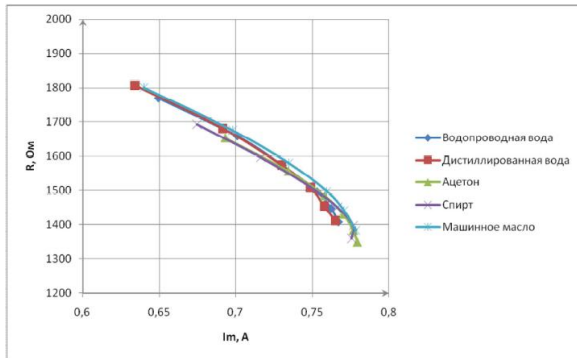
Рисунок 6 – Зависимость активного сопротивления механической ветви от тока механической ветви
