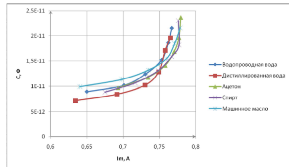
Рисунок 8 – Зависимость емкости механической ветви от тока механической ветви
