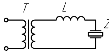
Рисунок 1 – Схема согласования УЗКС с выходом электронного генератора
