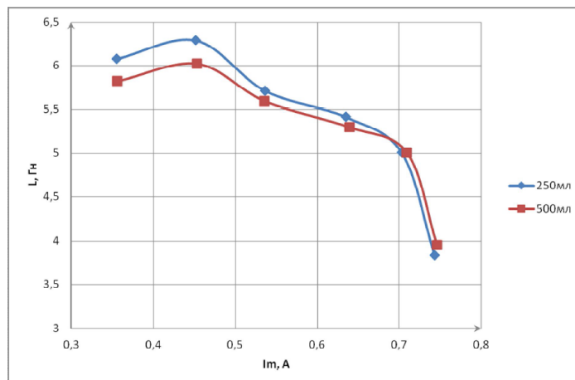
Рисунок 10 – Зависимость индуктивности механической ветви от тока механической ветви
