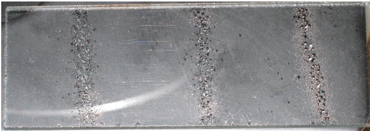
Рисунок 3 – Фотография следов распыляемого масла на стекле
