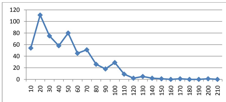
Рисунок 7 – Распределение частиц при использовании колебательной системы с частотой 60 кГц и распылительной иглы с рабочим окончанием в виде внутреннего конуса
