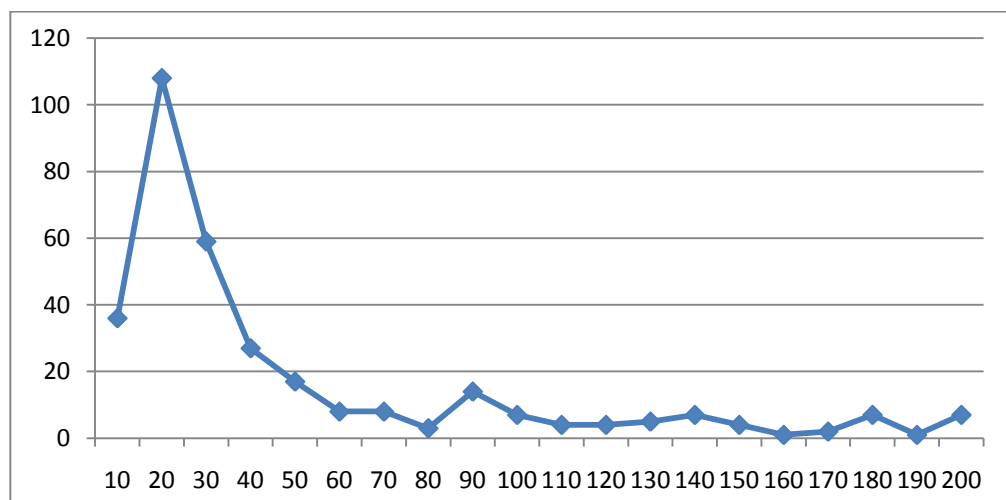
Рисунок 5 – Распределение частиц при использовании колебательной системы с частотой 22 кГц и распылительной иглы с рабочим окончанием в виде среза
