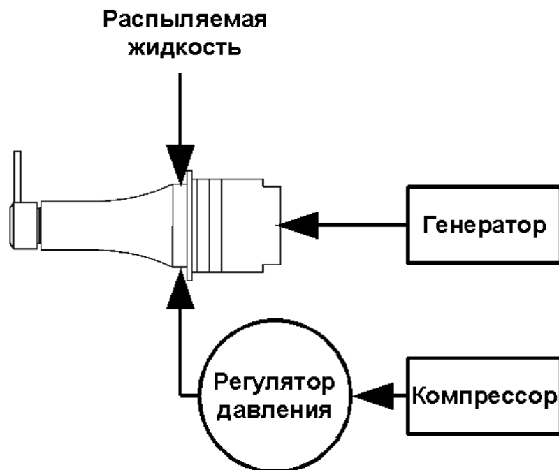
Рисунок 2 – Схема стэнда для исследования процесса распыления
