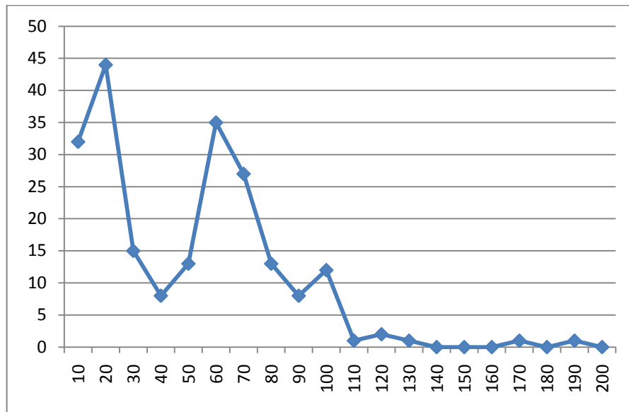
Рисунок 4 - Распределение частиц при использовании колебательной системы с частотой 60 кГц и распылительной иглы с рабочим окончанием в виде среза
