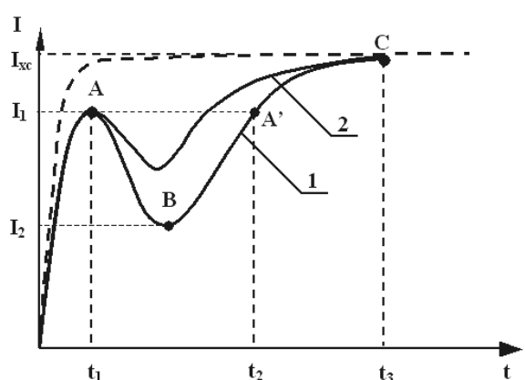
Рисунок 1 - Зависимость амплитуды тока, протекающего через пьезокерамические элементы ультразвукового излучателя в процессе формирования сварного шва
