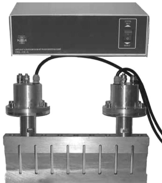
Рисунок 9 – Ультразвуковой аппарат для шовно-шаговой сварки термопластов.
