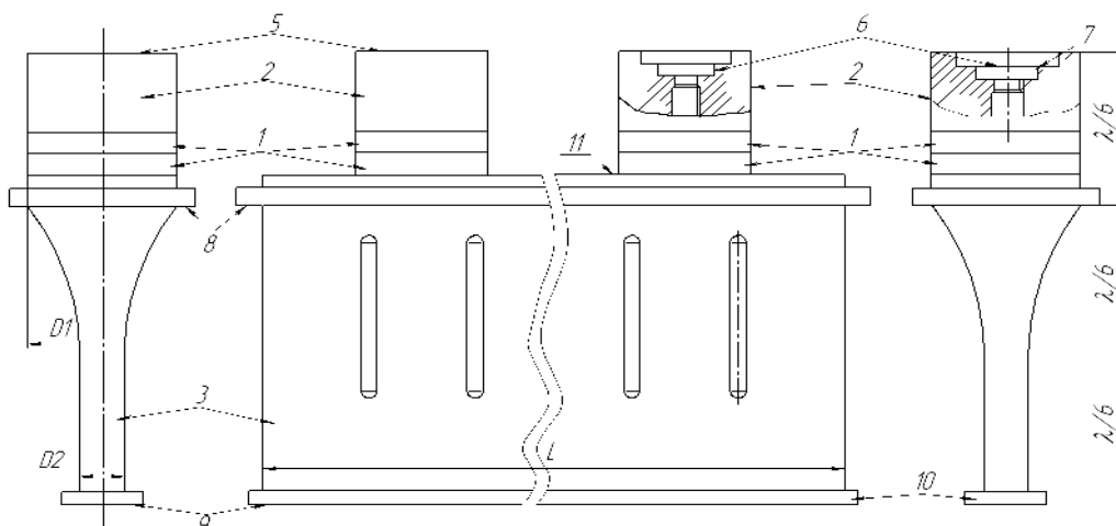
Рисунок 6 – Полуволновая пьезоэлектрическая УЗ колебательная система для выполнения протяженного шва.
