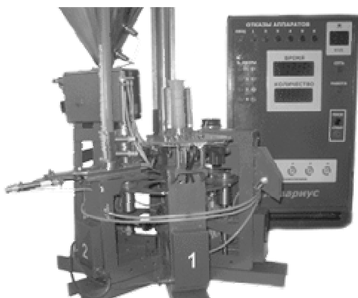
Рисунок 11 – Автоматизированная линия «Аквариус» производства картриджей для очистки воды.
