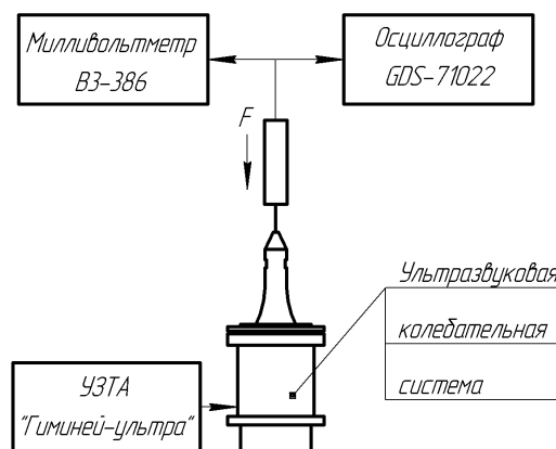
Рисунок 5 – Стенд для калибровки пьезоэлектрического приемного преобразователя.
