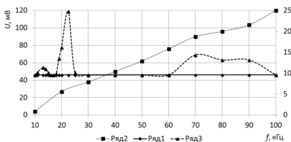
Рисунок 4 – Амплитудно-частотная характеристика пьезоэлектрического приемного преобразователя с пьезоэлементом 5 \times 5 \times 1 мм: на согласующем устройстве (ряд 2), с помощью пьезопластины (ряд 3), обработанная (ряд 1).
