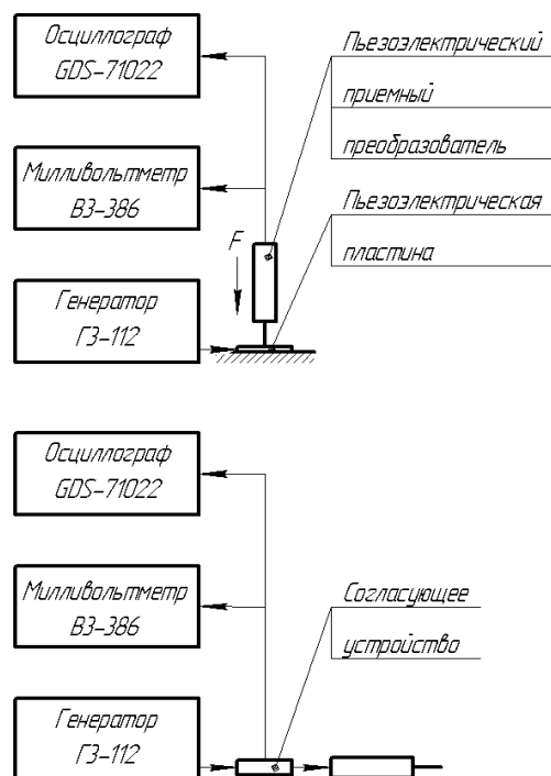
Рисунок 2 – Структурная схема стенда для измерения амплитудно-частотной характеристики.
