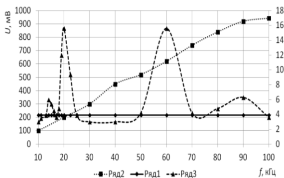
Рисунок 3 – Амплитудно-частотная характеристика пьезоэлектрического приемного преобразователя с пьезоэлементом \varnothing 7 \times 1 мм: на согласующем устройстве (ряд 2), с помощью пьезопластины (ряд 3), обработанная (ряд 1).
