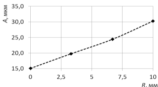
Рисунок 7 – Распределение амплитуды колебаний по излучающей поверхности рабочего инструмента ультразвукового технологического аппарата «Алена».
