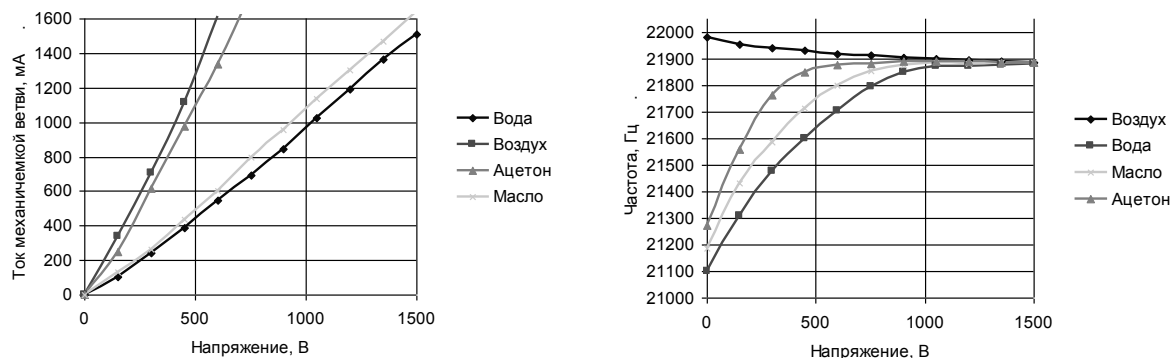
Рисунок 4 – Зависимости тока механической ветви и резонансной частоты колебательной системы от напряжения на пьезокерамических элементах ультразвуковой колебательной системы при использовании при использовании грибовидного рабочего инструмента диаметром 25 мм
