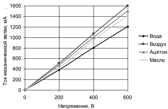
Рисунок 3 - Зависимости тока механической ветви и резонансной частоты колебательной системы от напряжения на пьезокерамических элементах ультразвуковой колебательной системы при использовании цилиндрических инструментов.
