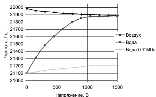
Рисунок 5 - Зависимость резонансной частоты от напряжения питания УЗКС
