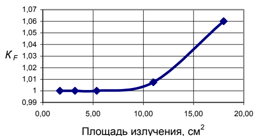
Рисунок 7 – Зависимость коэффициента K_F от площади поверхности излучения
