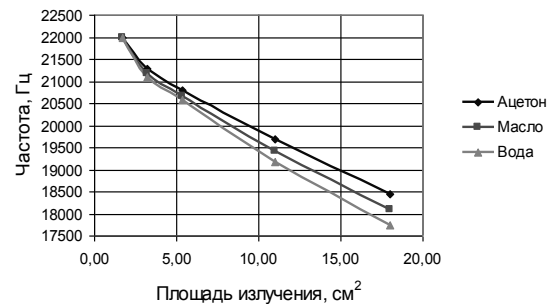
Рисунок 6 – Расчетная зависимость резонансной частоты колебательной системы от площади поверхности излучения
