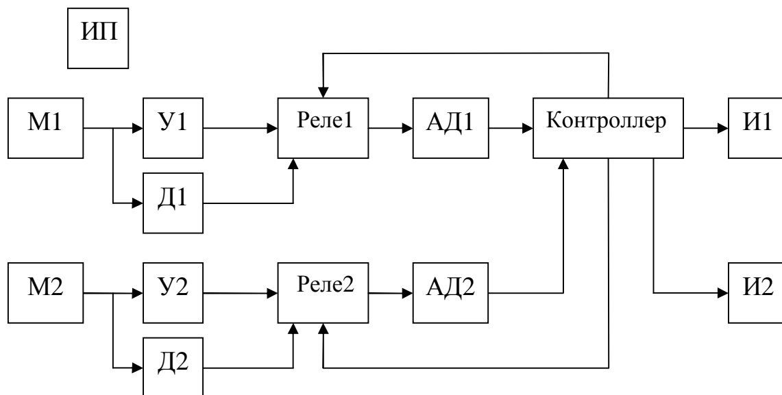
ИП – источник питания; М1, М2 – микрофоны первого и второго каналов; У1, У2 – усилители; Д1, Д2 – делители; АД1, АД2 – амплитудные детекторы; И1, И2 – индикаторы
