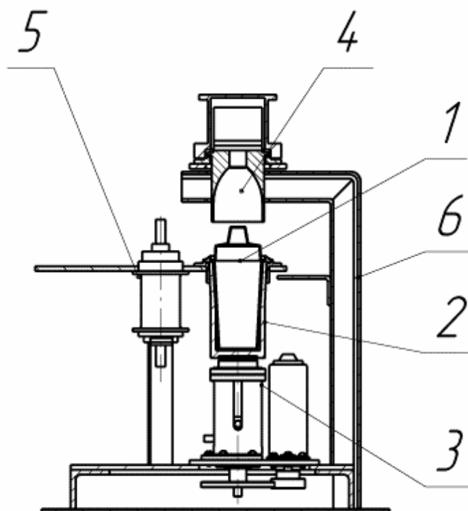
Рисунок 3 Установка для сварки элементов картриджа.
