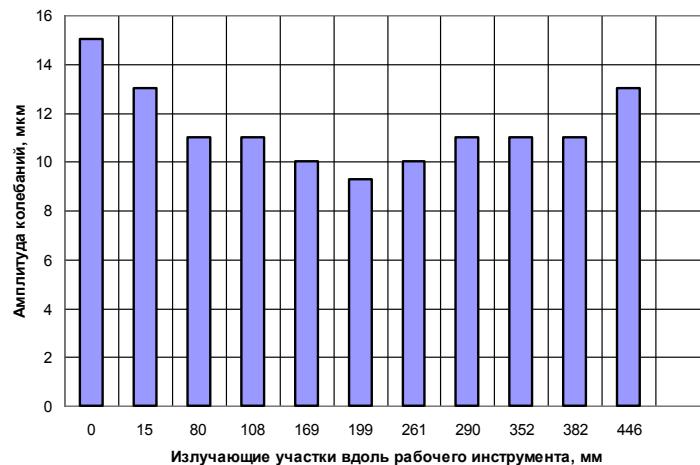
Рисунок 6 – Распределение амплитуды колебаний излучающих поверхностей инструмента ВДОЛЬ ОСИ
