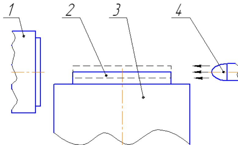
Рисунок 4 – Схема стенда для измерения амплитуды колебаний, где 1 - окуляр микроскопа, 2 – торец ультразвуковой колебательной системы, 3 – технологический объем с жидкостью, 4 – стробоскопическая система освещения
