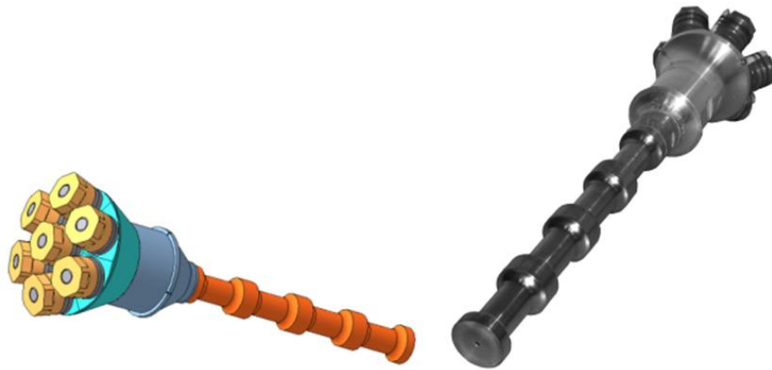
Рисунок 3 – Многополуволновая ультразвуковая колебательная система
