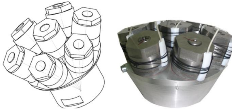
Рисунок 2 – Конструктивные схемы многопакетных преобразователей
