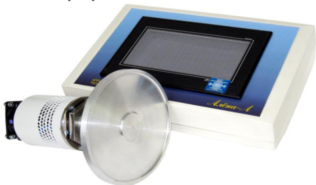
Рис. 2. Ультразвуковой генератор с дисковым излучателем для сушки волос.
